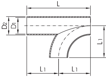
tee bends SSS
